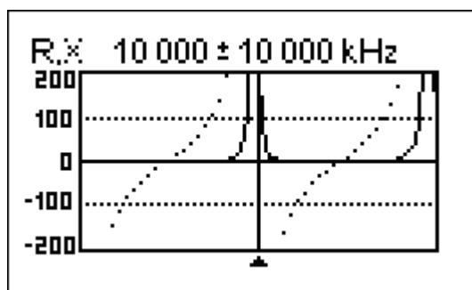
Offenes Kabel
