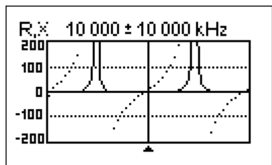
Kurzgeschlossenes Kabel
