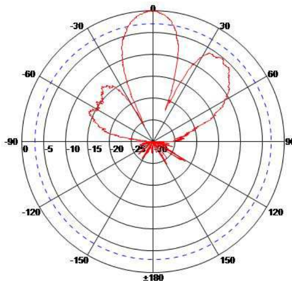
5 GHz E-Plane
