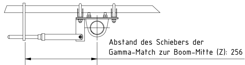
A-A (1:8)
