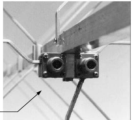
Bild 2 X-Quad Anschlußkasten
