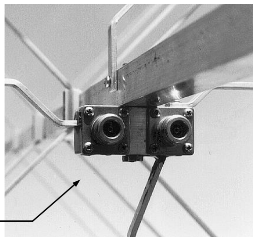
Bild 2 X-Quad Anschlußkasten
