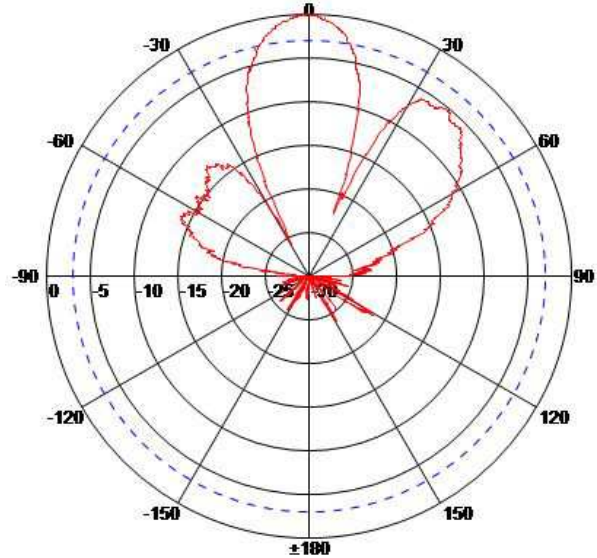
5 GHz E-Plane
