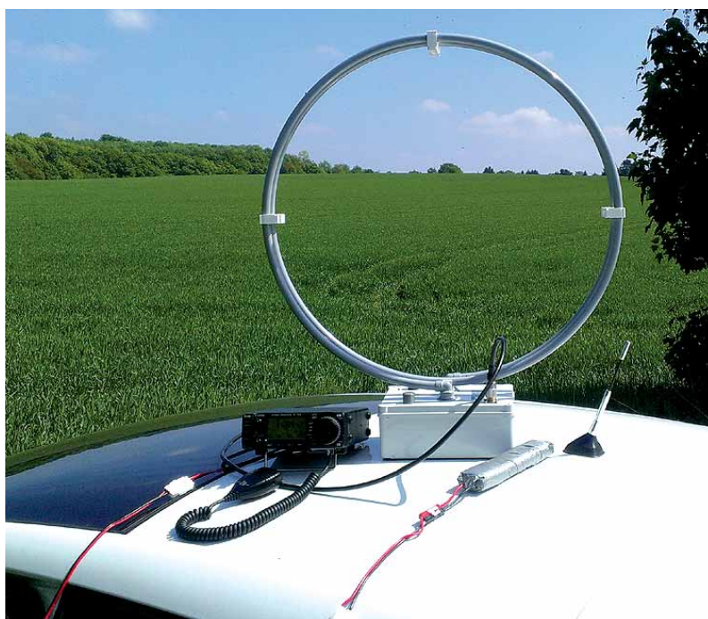
Bild 5: Testaufbau Outdoor
