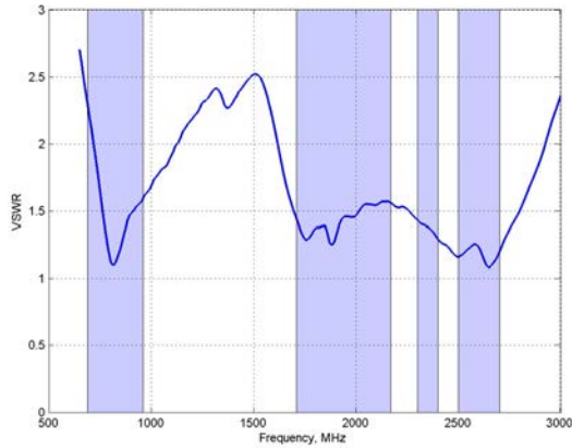
VSWR
